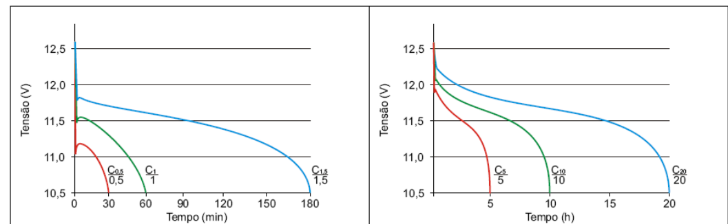
Curvas características de descarga a 25°C
